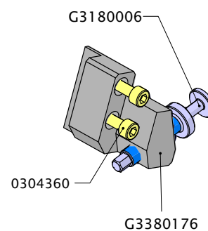
G2920723 CODICE DEL GRUPPO ASSEMBLY CODE PER/FOR (3"3/4)
