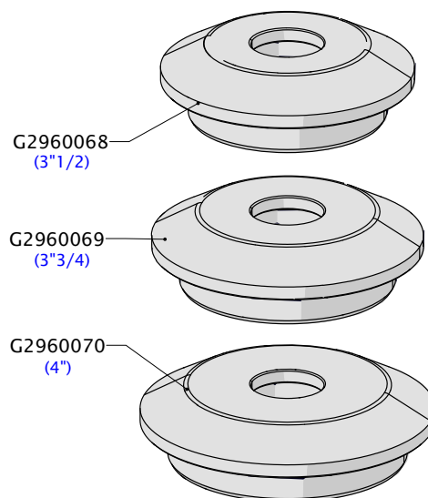
CALIBRI ORRIZZONTALE BORDO BOARD HORIZONTAL GAUGES
