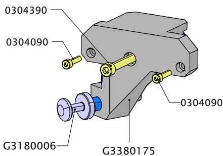
G2920605 CODICE DEL GRUPPO ASSEMBLY CODE PER/FOR (4")
