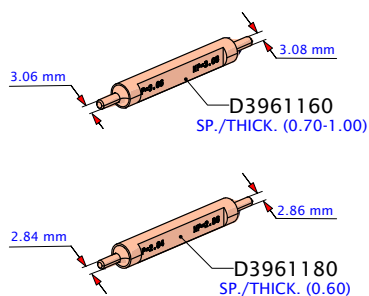
CALIBRI PASSAGGIO AGHI GAUGES PASSAGE NEEDLES
