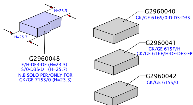
CALIBRI CONTROLLO PLATORELLO DIAL CONTROL GAUGES
